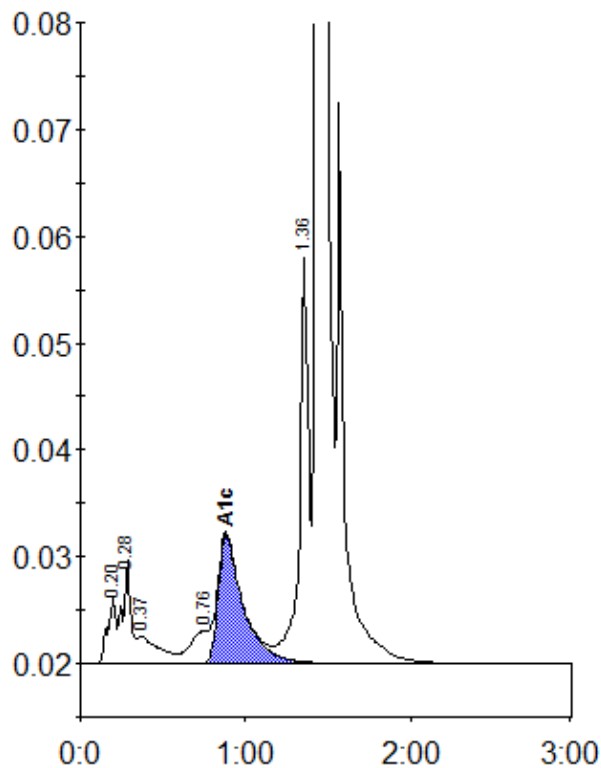
Peak table - ID: 10248164
